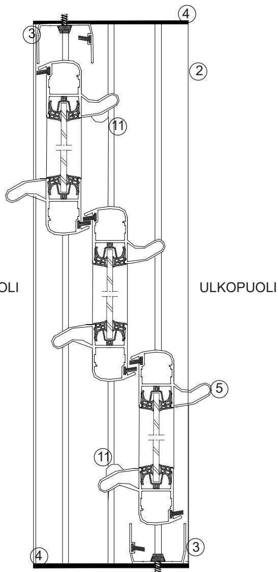
3-osainen peilikuva liukuovielementti (yläpuolelta katsottuna)
