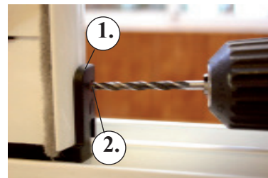
Liukuovia/-ikkunoita irrotettaessa lukitustappi (2) porataan ulos ja lukkopala (1) irrotetaan, minkä jälkeen liukuovet/-ikkunat voi nostaa pois.
