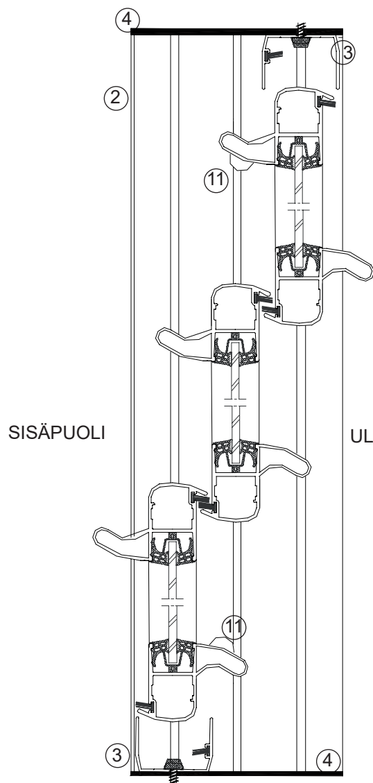
3-osainen oletussuuntainen liukuovielementti (yläpuolelta katsottuna)
